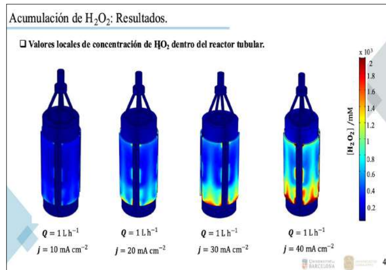
Imágenes: Creación de un modelo CFD para el cambio de escala de un reactor 3D
