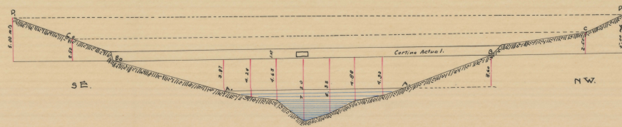
PERFIL DE LA CORTINA ESCALA 1:150 VERT. Y HOR.
