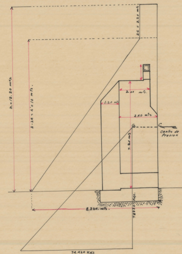
CORTE DE LA CORTINA. ESC 1:100
